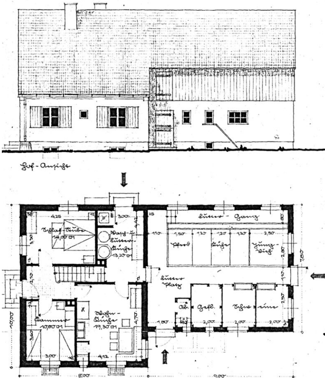
Entwurf für ein kombiniertes Wohn- und Stallgebäude auf Neubauernland, 1946.
